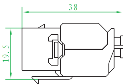
BOČNÍ POHLEDY
