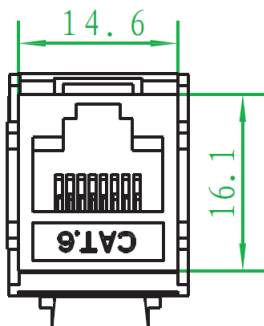
PŘEDNÍ POHLED
