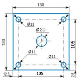
príruba KS-M
