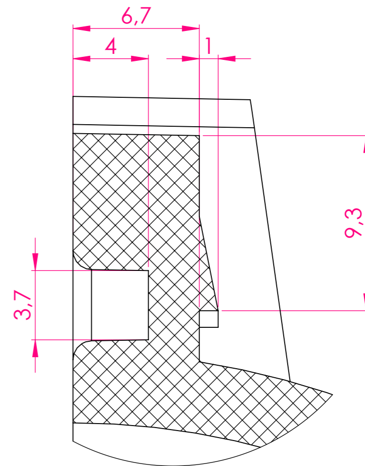
DETAIL D MĚŘITKO 5 : 1
